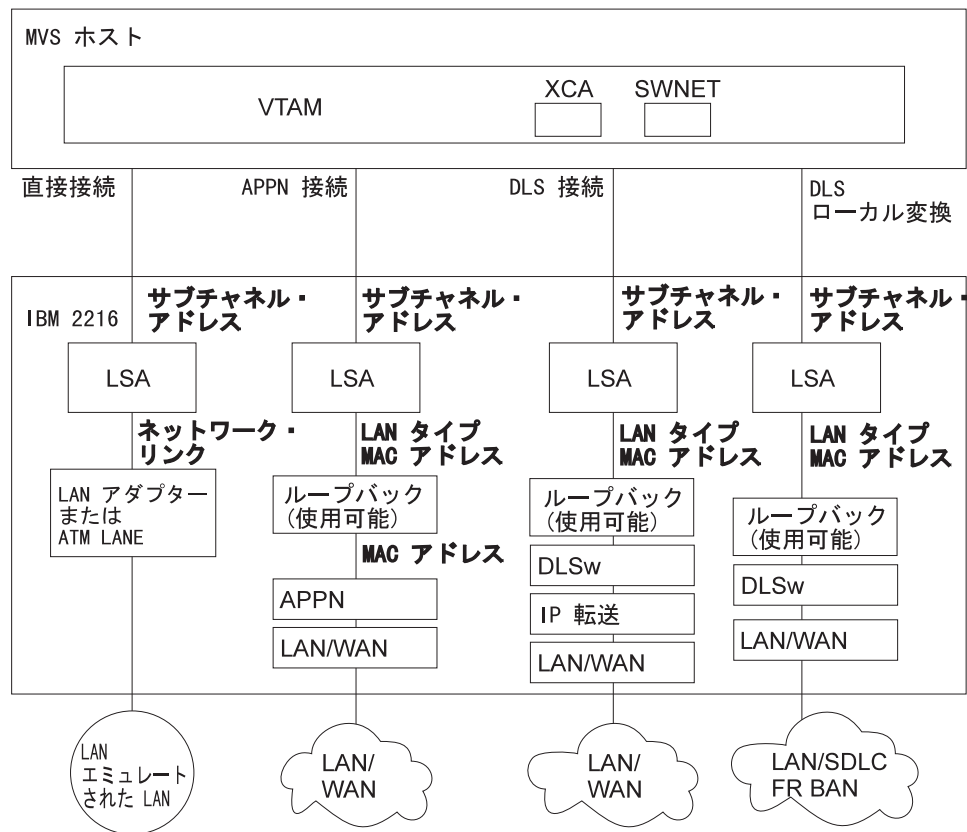
図26. リンク・サービス・アーキテクチャ (LSA) バーチャル・ネットワーク・ハンドラーの構成
