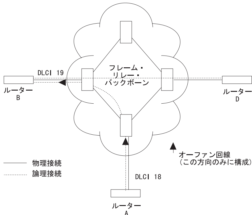
図40. オーファン回線
