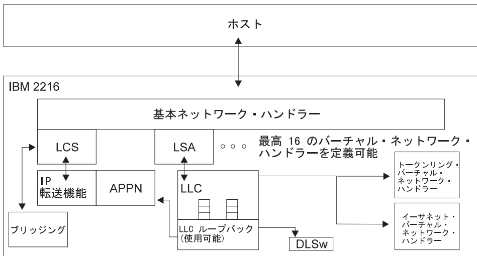
図 23. LCS および LSA の場合の 2216 バーチャル・ネットワーク・ハンドラー
