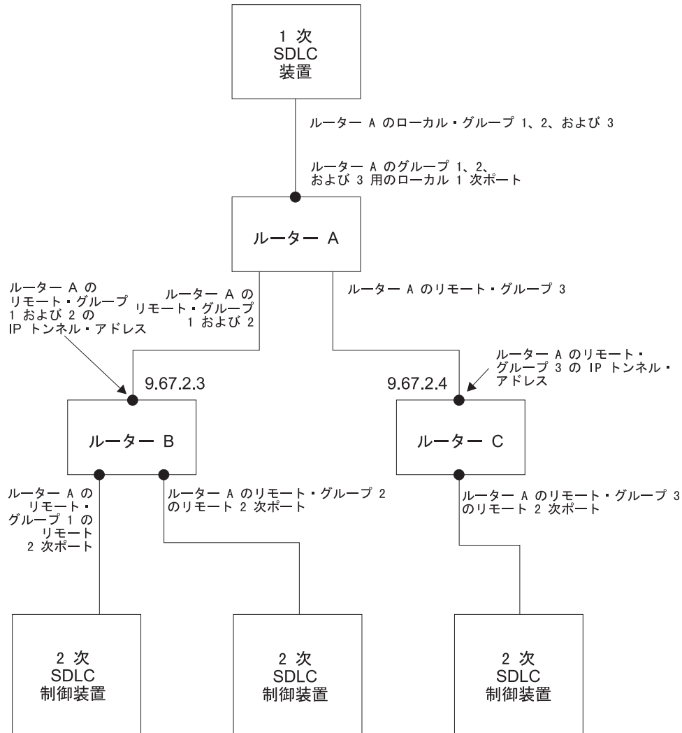
図 47. SDLC リレー構成の例
