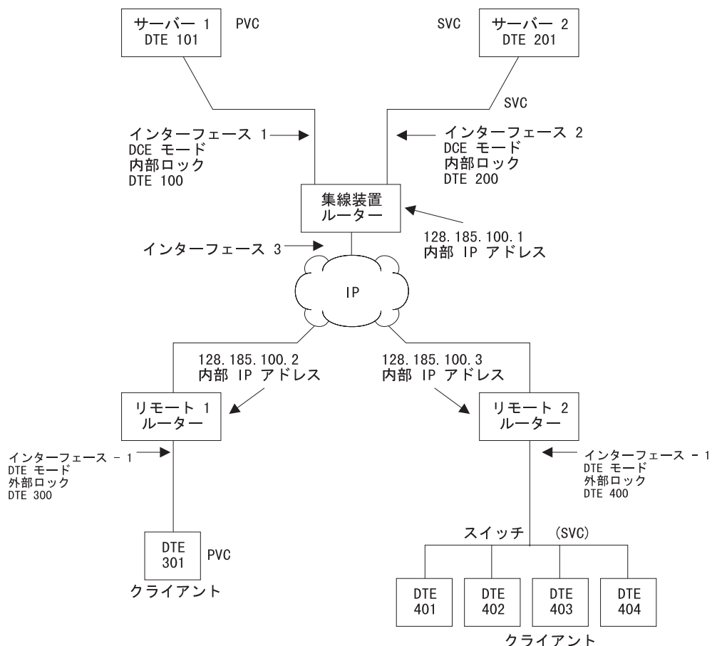
図 37. XTP 構成例
