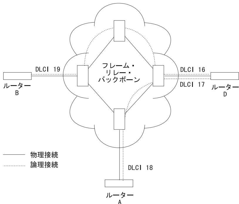
図38. フレーム・リレー・ネットワーク内の DLCI
