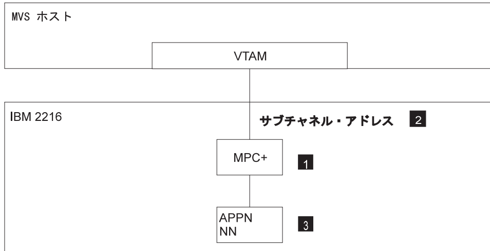
図32. マルチパス・チャネル+ (MPC+) を介する APPN 用のバーチャル・ネットワーク・ハンドラーの構成
