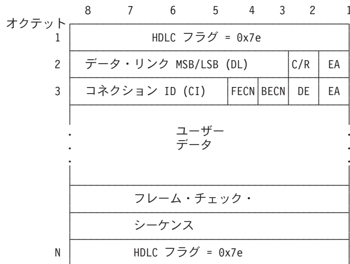
図41. フレーム・リレーのフレーム・フォーマット
