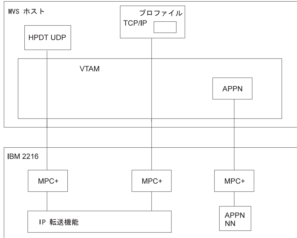
図 31. さまざまなタイプの MPC+ 接続.
